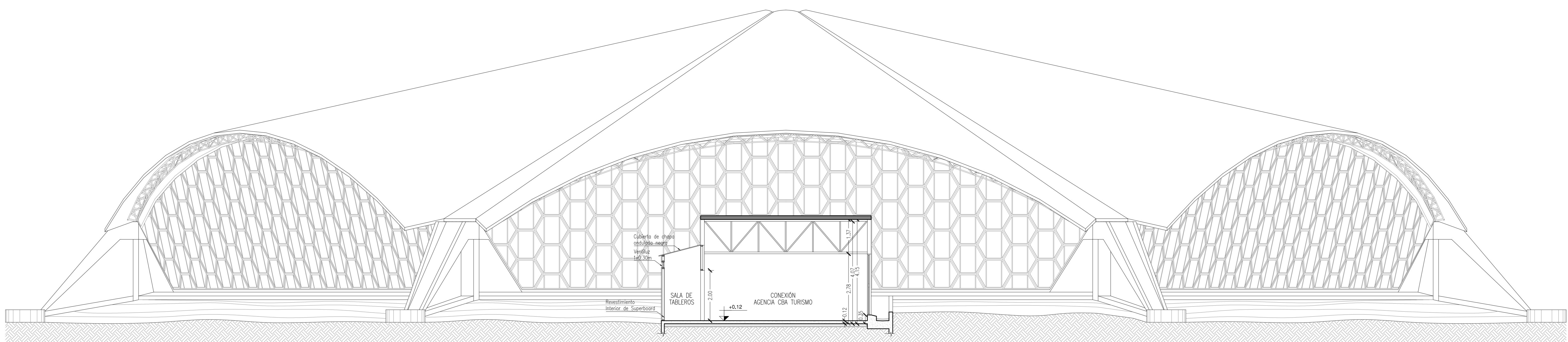
CORTE C-C
