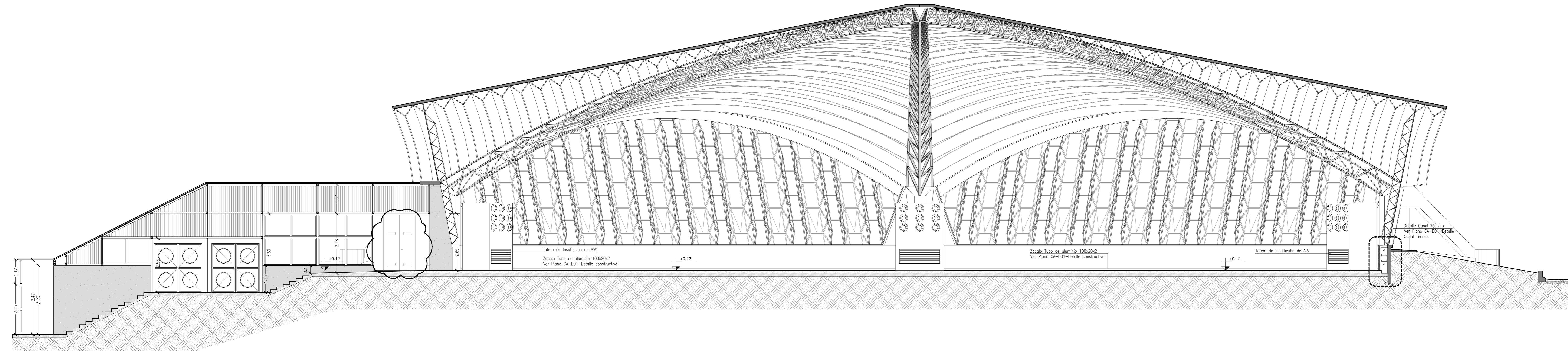
CORTE B-B
